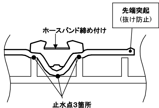
図4. リブ管取付概略図
