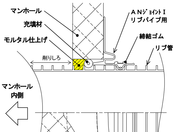
図3. リブ管への取り付け概略図
