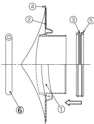
図2. 製品仕様図
